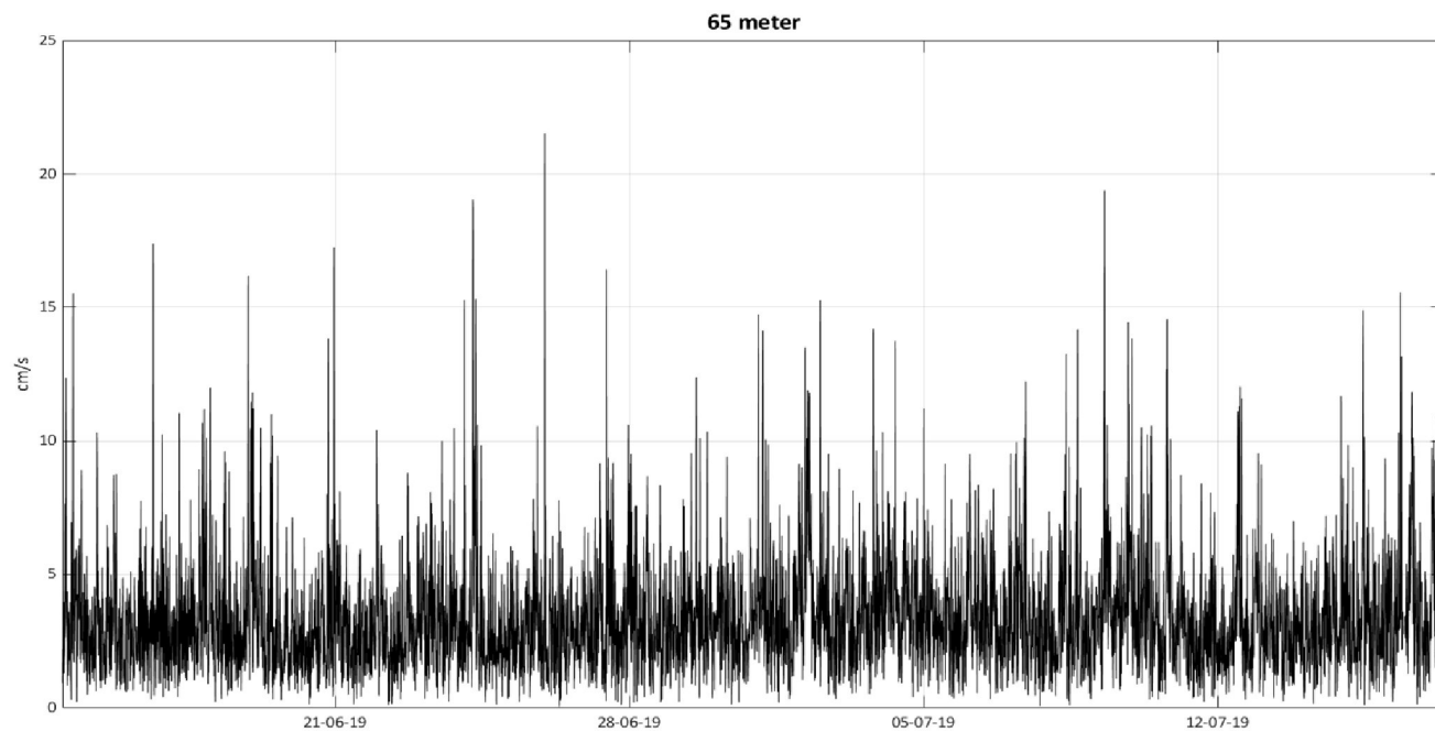
Figur 3: Vannstrømshastighet (cm/s) på 65 meters dyp ved Klubben i perioden 14.06.–17.07.2019.
