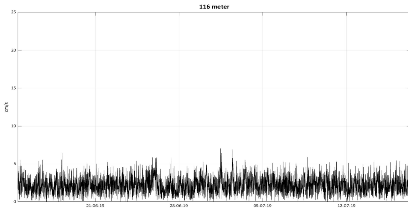
Figur 4: Vannstrømshastighet (cm/s) på 116 meters dyp ved Klubben i perioden 14.06.–17.07.2019.
